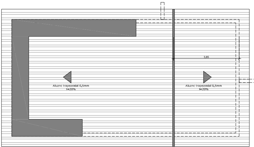
COBERTURA ESC. 1/50
